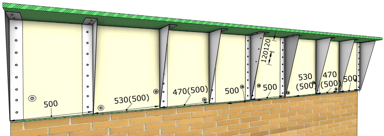
Abb. 24: Perspektivische Ansicht zwei zusammengefügter Dachrandelemente, beim Stoss ist ein Stützblech gespiegelt auszubilden und mit drei metrischen M8-Schrauben oder drei Popnieten 4,8 x 8 mm zu verbinden. Masse in mm.
